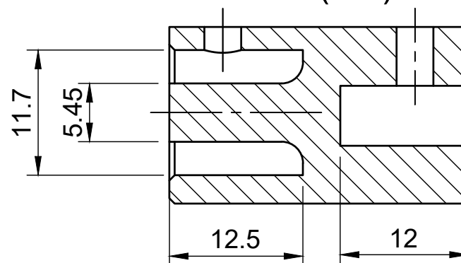
A-A (2:1)
